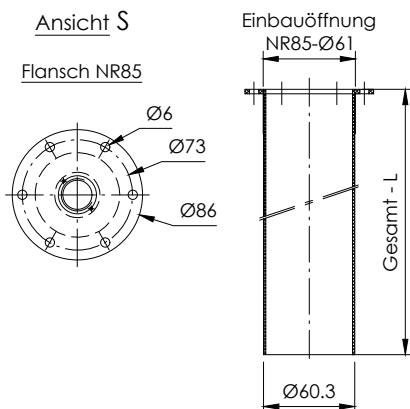
Darstellung Schutzrohr
