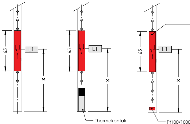
04 04 + Thermokontakt 04 + Pt 100/1000
