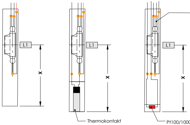
02 02 + Thermokontakt 02 + Pt100/1000
